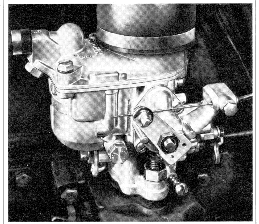
CARBURATEUR INVERSÉ
