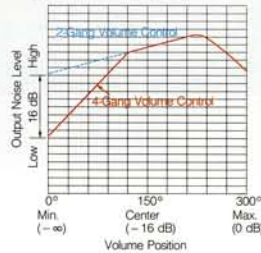
Ausgangsrauschen (4- und 2-stufiger Lautstärkereger)
