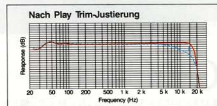
Effekt der Play Trim-Justierung
