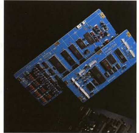
DSP-Schaltplatine
