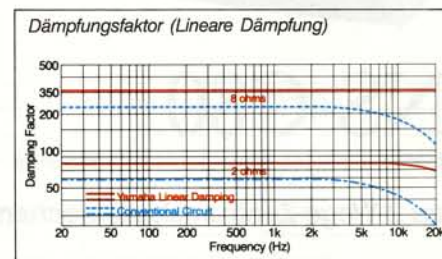
Die erweiterte Linearität des Dämpfungsfaktors sorgt auch bei Frequenzen zwischen 10 und 20 kHz, wo gewöhnlich Pegelabnahmen auftreten, für einen hohen stabilen Dämpfungsfaktor. Die Folge ist eine klare und exakte Wiedergabe im gesamten Signalbereich.
