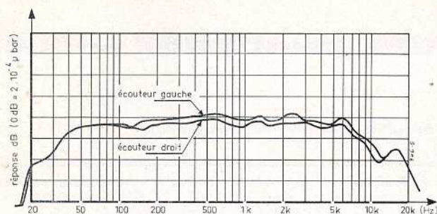
Fig. 6. — Courbes de réponse d'une paire stéréophonique d'écouteurs électrostatiques « Koss-ESP-6 », après mise au point d'un coupleur, ou oreille artificielle, convenant aux fréquences supérieures à 8 kHz.
