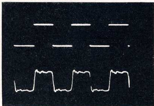
Fig. 7. — Réponse d'un écouteur « Koss-ESP-6 » à un signal carré à 400 Hz. Le tracé supérieur donne le signal incident aux bornes de l'écouteur ; au-dessous la réponse du transducteur acoustique.
