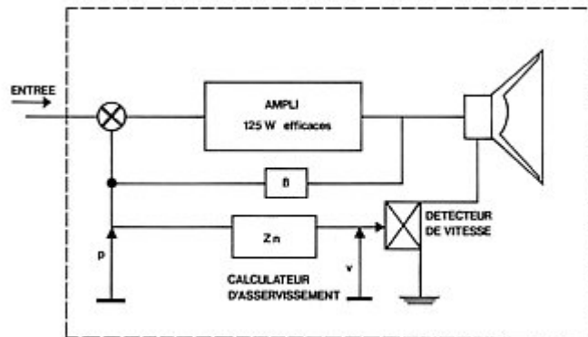
Fig. V.6 Principe de l'asservissement de pression
