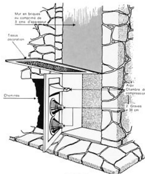
Fig. III.1 Une magnifique installation : un immense placard de part et d'autre d'une cheminée. Chaque enceinte contient 2 \times 38 \text{ cm} pour les graves et une chambre de compression dans l'aigu.
