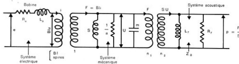
Fig. II.5 Analogie électrique du piston plat avec un baffle indéfini.
