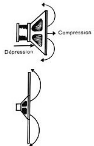
Fig. II.3 L'onde arrière réagit sur l'onde avant
