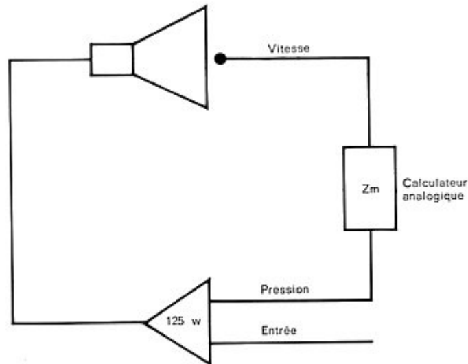
Fig. V.9 Le système APF 3a d'asservissement de pression
