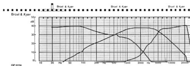
Fig. II.6 Filtre de l'Arioso 3a
