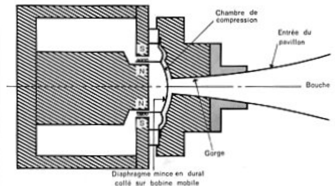
Fig. III.10 Haut-parleur à chambre de compression d'extrême aigu
