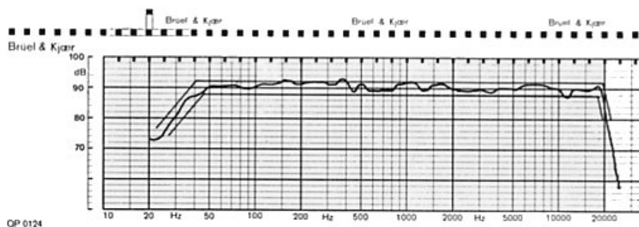
Fig. I.3 Courbe de réponse de l'Andante 3a
