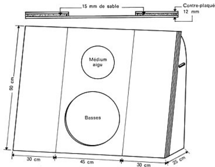
Fig. III.7 Un excellent baffle plan sablé
