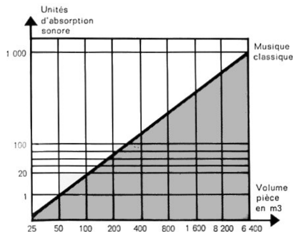
Fig IV.5 Unité d'absorption sonore fonction du volume de la pièce
