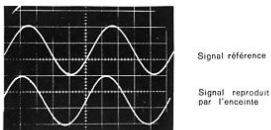
Fig. I.4 Distorsion harmonique de l'Arioso 3a
