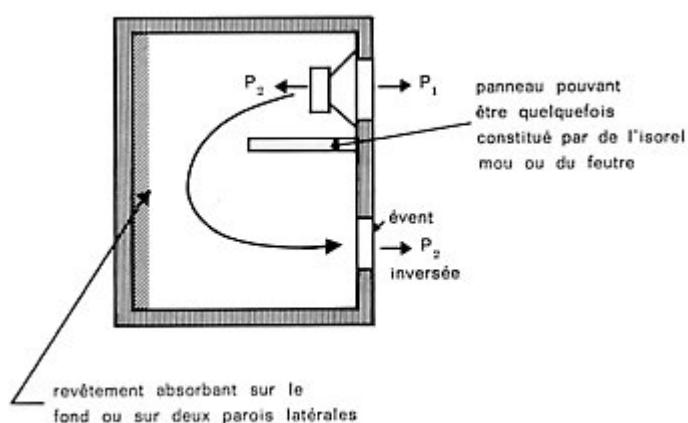
Fig. III.4 a Principe du meuble inverseur de phase (bass-reflex)
