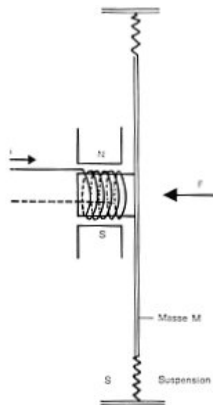
Fig. V.4 Schéma d'un haut-parleur plan
