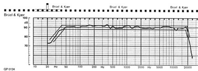
Fig. V.8 Courbe de réponse de l'andante 3a
