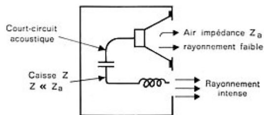
Fig. III.6 Comportement du bass-reflex à la fréquence de résonance du haut-parleur
