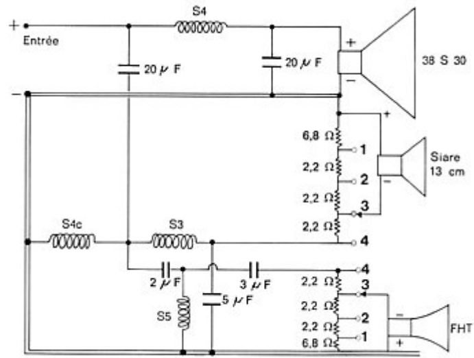
Fig. II.8 Schéma du filtre précédent
