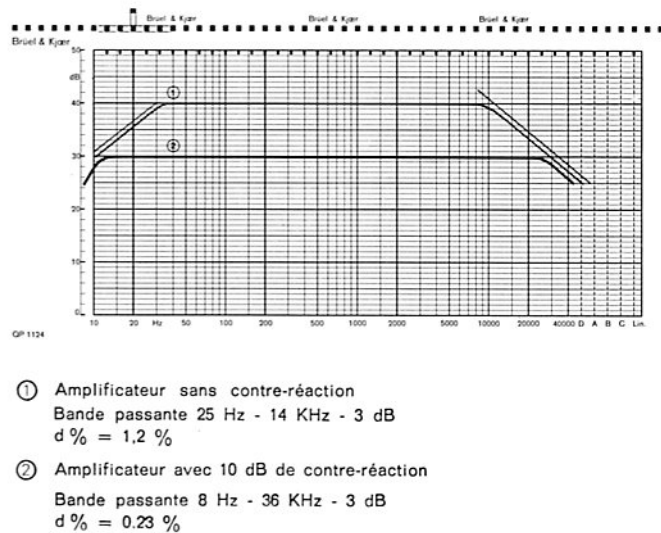
Fig. V.3 Amélioration de la bande passante par contre-réaction
