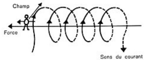
Fig. II.2 Principe du haut-parleur
