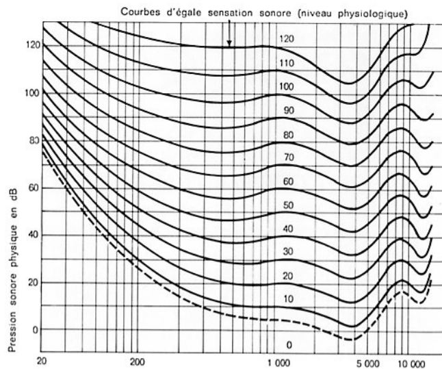
Fig. VI.2 Courbe de Fletcher Munson
