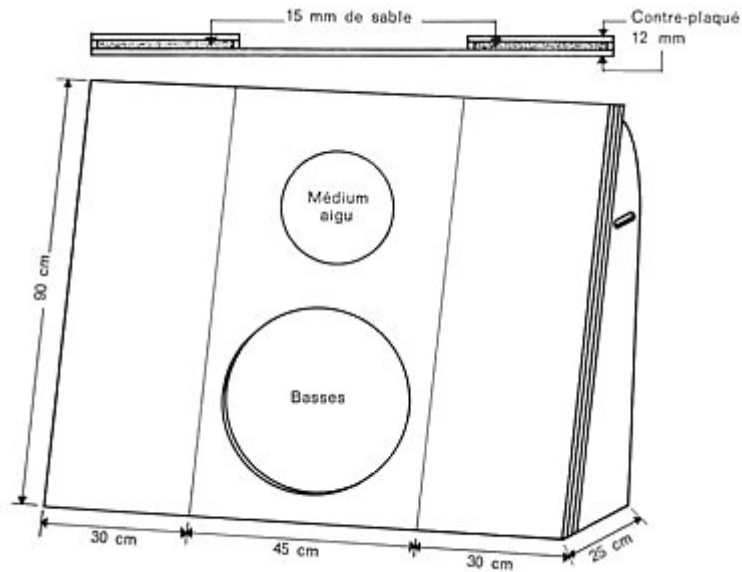
Fig. II.4 Un procédé simple permettant d'augmenter le trajet de l'onde arrière
