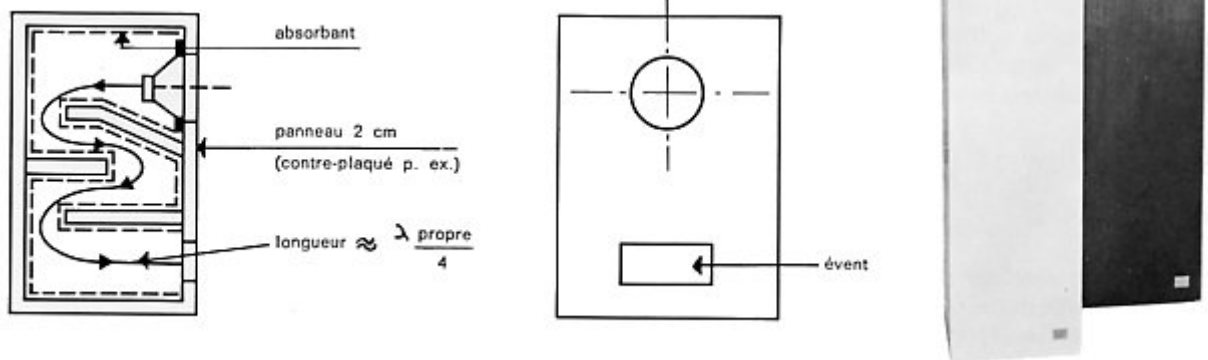
Fig. III.3 Principe du labyrinthe acoustique
