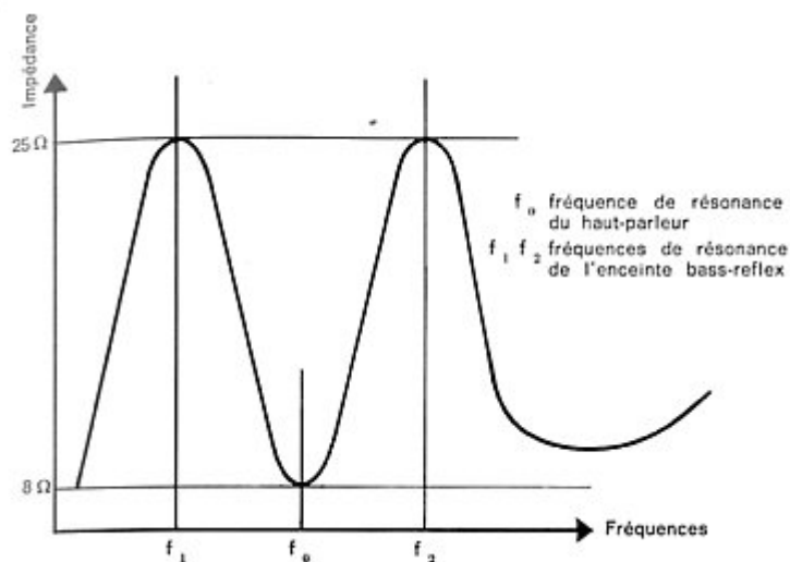
Fig. III.5 Courbe d'impédance du bass-reflex
