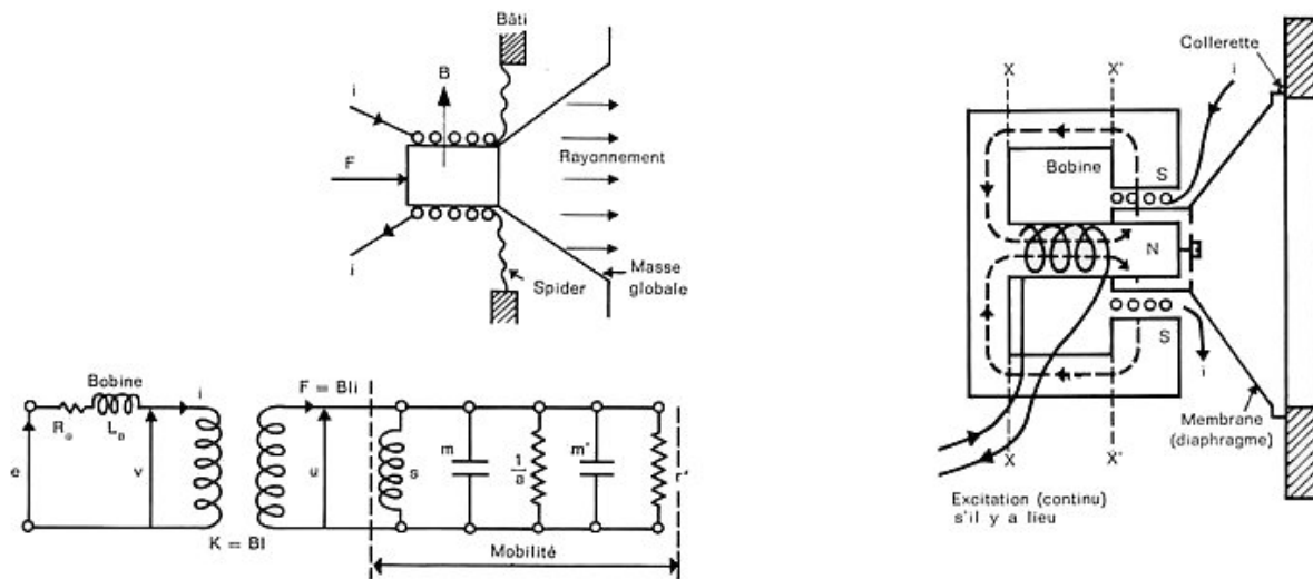
Fig II.1 Schéma équivalent du quadripôle haut-parleur
