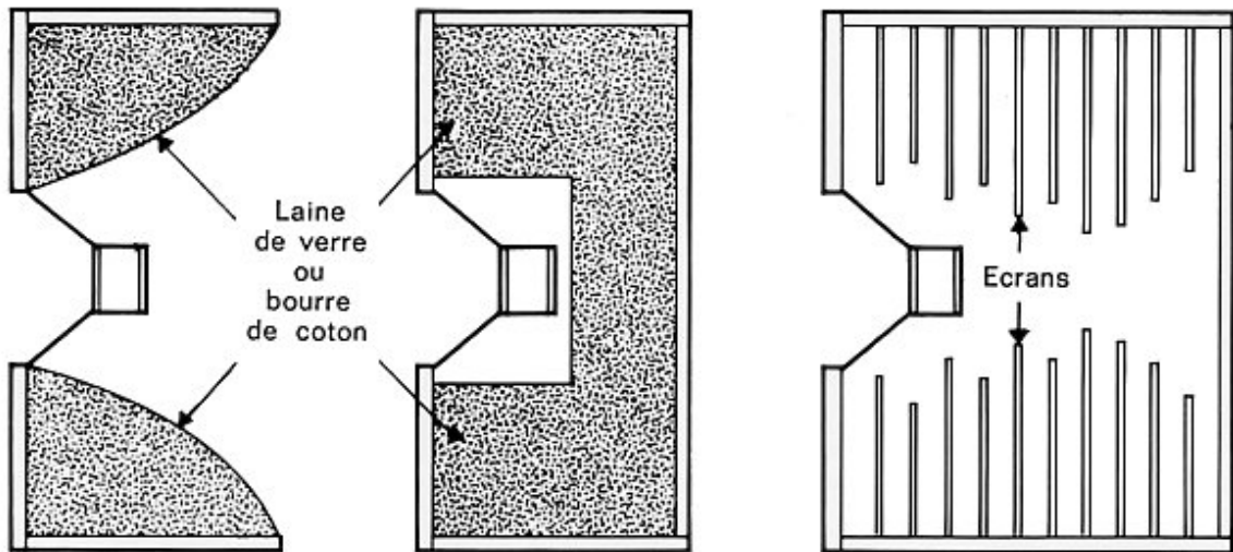
Fig. III.2 Trois version de coffret réalisant l'absorption de l'onde arrière de la membrane
