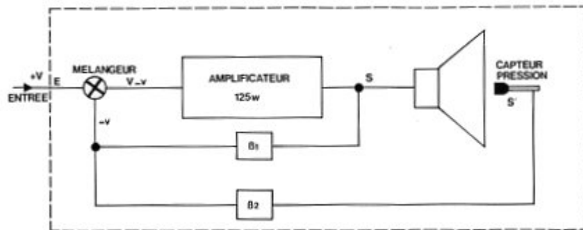
Fig. V.3 Contre-réaction appliquée à un système électro-acoustique
