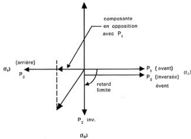
Fig. III.4 b Composition des pressions engendrées par le cône et l'évent
