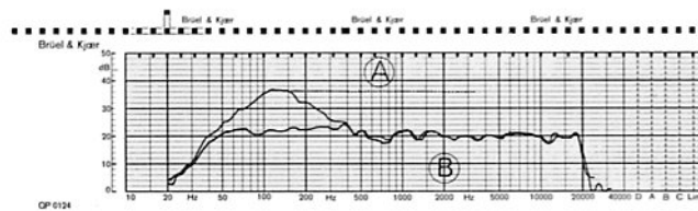
Fig. V.7 La courbe A est la réponse du haut-parleur sans asservissement. La courbe B, réponse de l'enceinte asservie.
