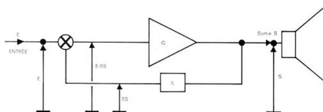
Fig. V.1 Amplificateur avec boucle de contre-réaction
